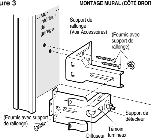
MONTAGE MURAL (CÔTÉ DROIT)
