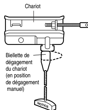
Position verrouillage (Position de dégagement manuel)
