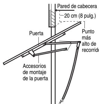
Puerta de una sola pieza sin riel guía: accesorios de montaje
