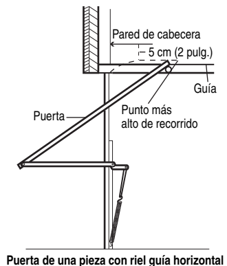
Puerta de una sola pieza con riel guía horizontal
