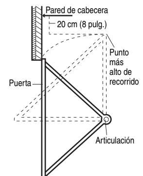
Puerta de una sola pieza sin riel guía: accesorios de articulación
